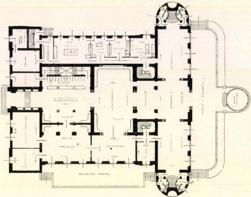
A gyógyterem földszinti alaprajza.
