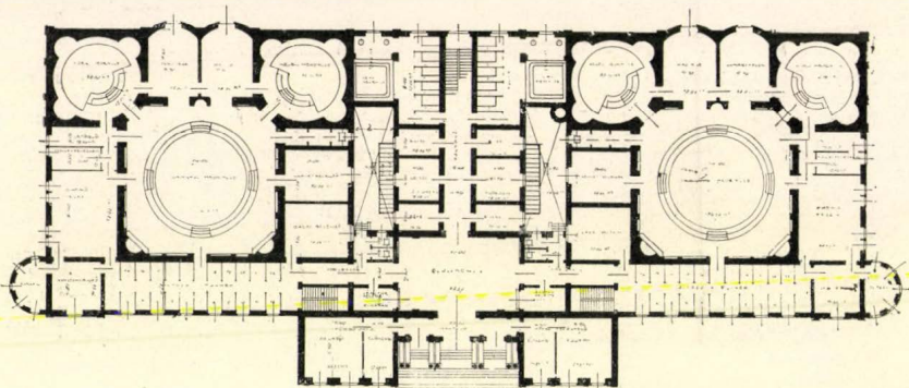
A meleg fürdő földszinti alaprajza.
