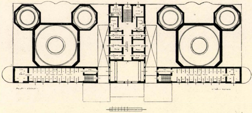
A meleg fürdő I. emeleti alaprajza.
